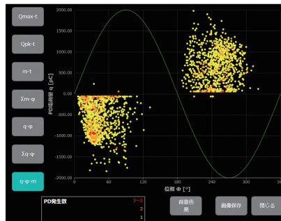
q-Φ-m解析圖表
