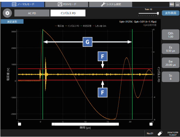
部分放電檢測的閾值與判斷區間的設定
