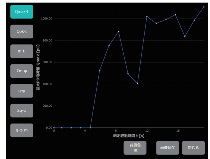
Qmax-t解析圖表
