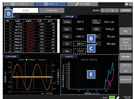
AC PD PDIV模式測量
