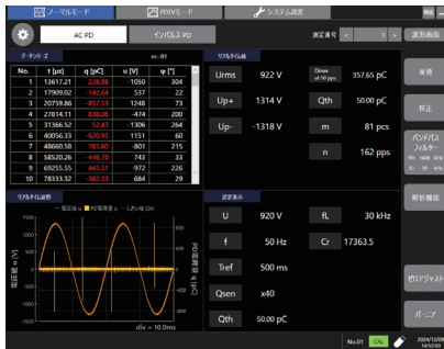
AC PD一般模式測量
