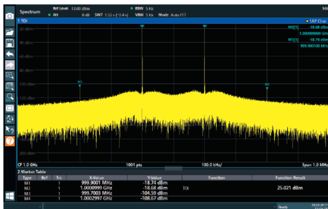
三階截止點 (TOI) 量測
