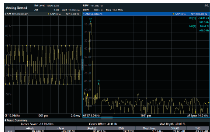
有關調幅訊號的 THD 量測：調變訊號的一次諧波得到很好的抑制 (74 dB)
