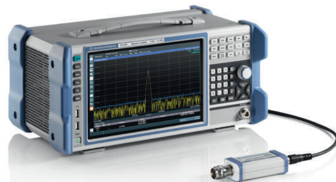
R&S®FPL1-K9 選配以及 R&S®NRP 功率探棒將 R&S®FPL1000 轉換為功率計
