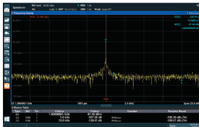
標記功能實現簡單的相位雜訊量測
