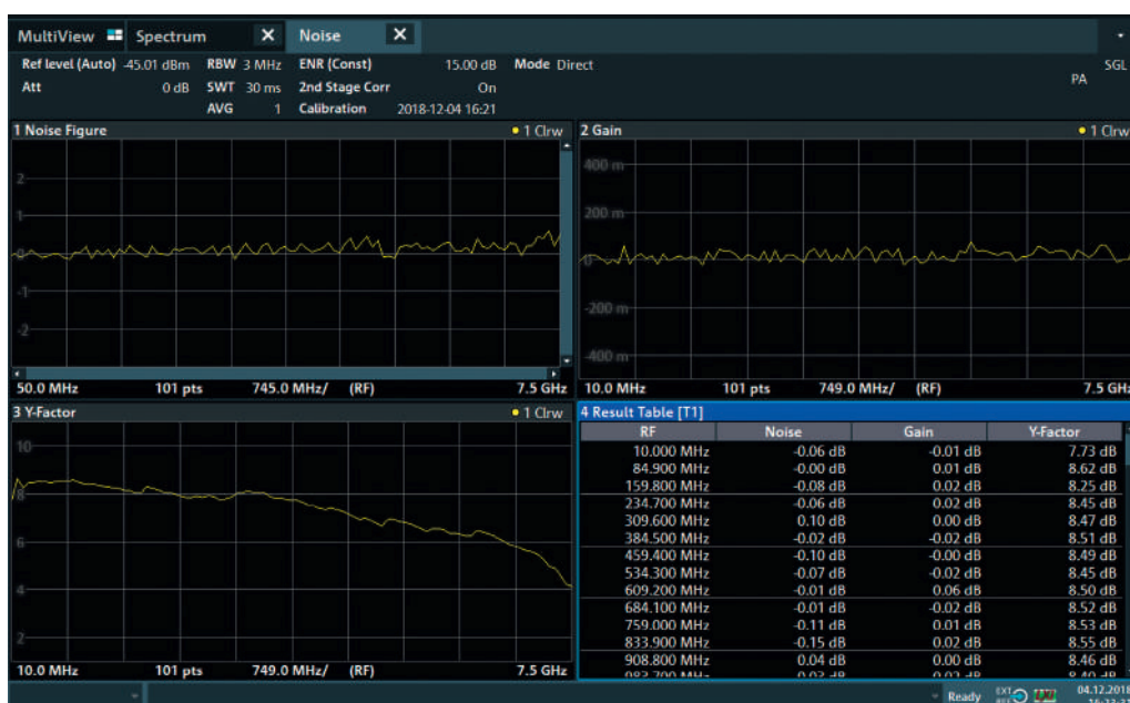
雜訊係數、增益及 Y 因子與頻率的同步視圖，以及數值形式的結果表
