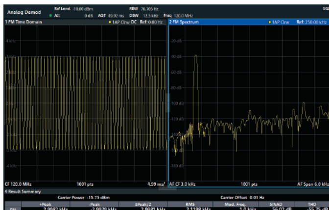
顯示調變訊號及其頻譜、峰值和 RMS 偏差
