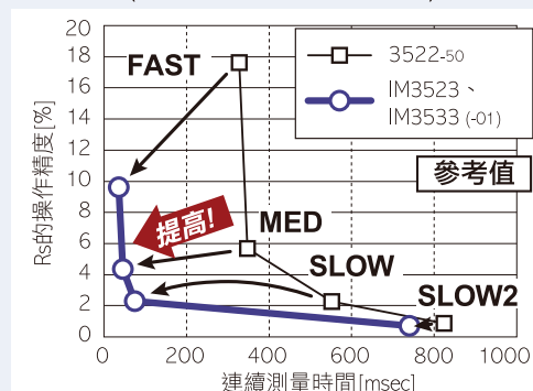
C-D, ESR測量(100kHz)的連續測量時的連續測量時間和Rs的操作精度 (取樣速率: 鋁制電解電容器1.5 \mu F)
