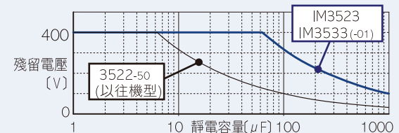
能夠保護 LCR 測試儀的靜電容量和殘留電壓的關係
