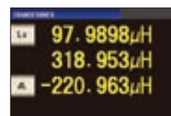
變壓器測量模式 電感差測量介面
